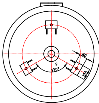
支座方位图
